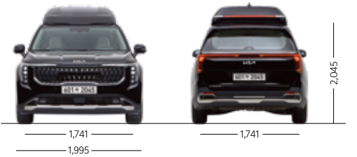
※ 가솔린 19인치 타이어 기준, 단위 : mm
